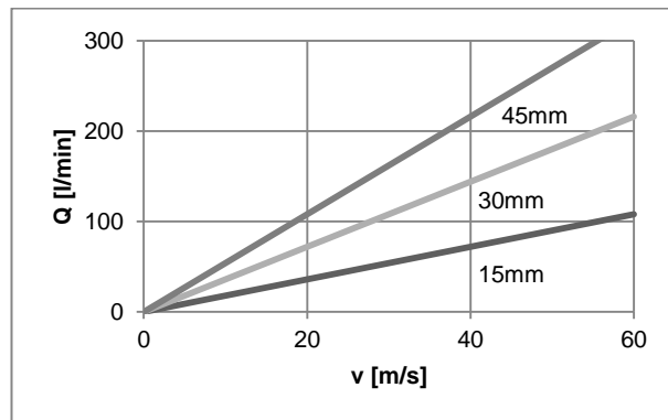
Abbildung 3: Erforderlicher Kühlmittelmengen für verschiedene Schleifscheibendicken in Abhängigkeit der Umfangsgeschwindigkeit. (Strahlhöhe: 2 mm)
